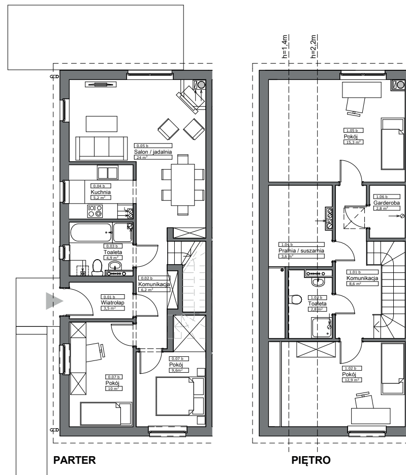
Plan pomieszczeń
